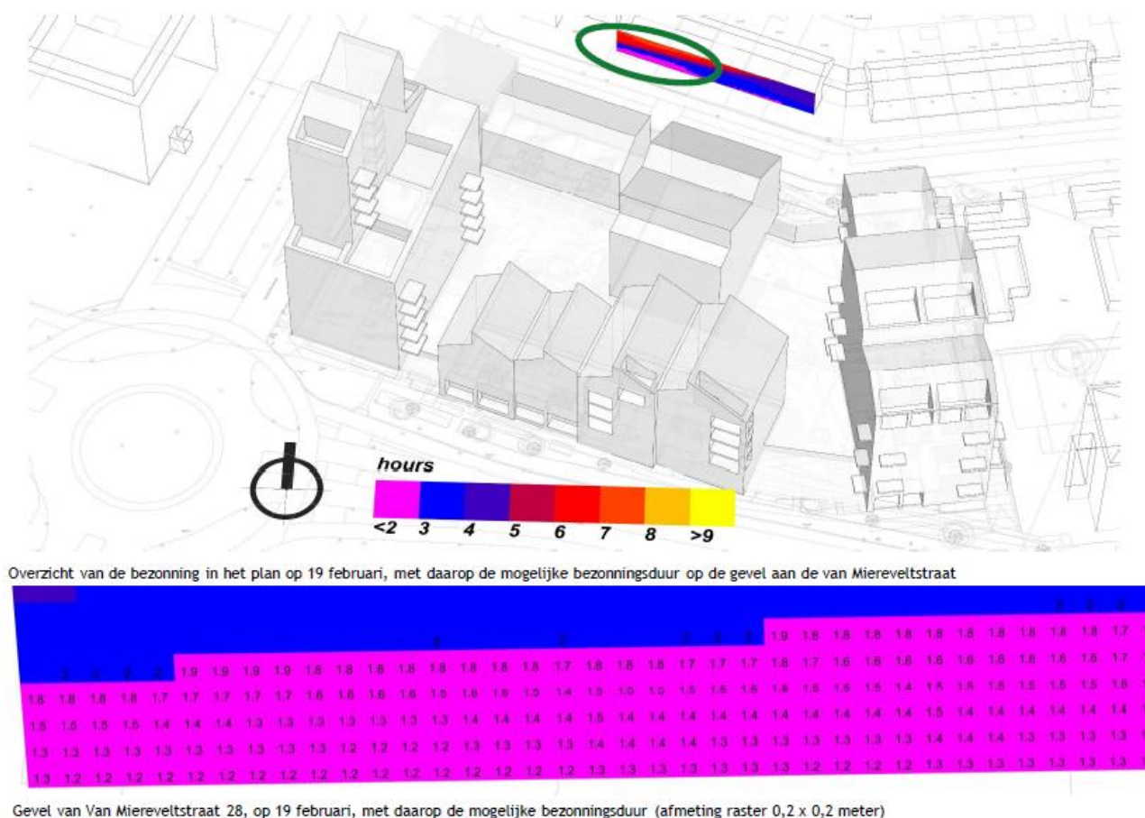
Figuur 14: Overzicht van de bezonning op de gevels van de woningen aan de Van Miereveltstraat
